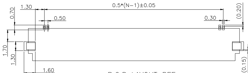
P.C.B LAYOUT REF
