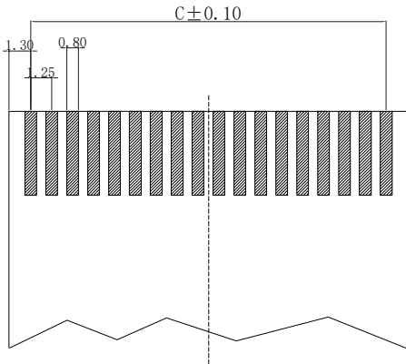
适用电缆(proper cable) (δ=0.3±0.02mm)
