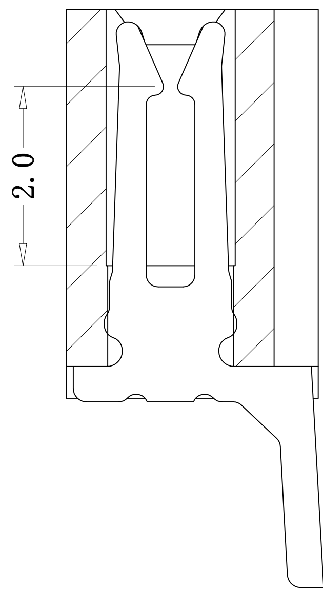
SECTION A-A
