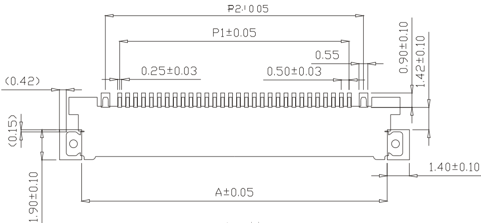
P.C.B LAYOUT
