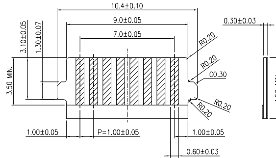
FFC SPEC 公差: ±0.05
