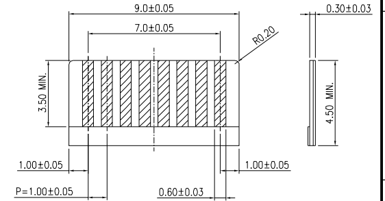
FFC SPEC 公差: ±0.05
