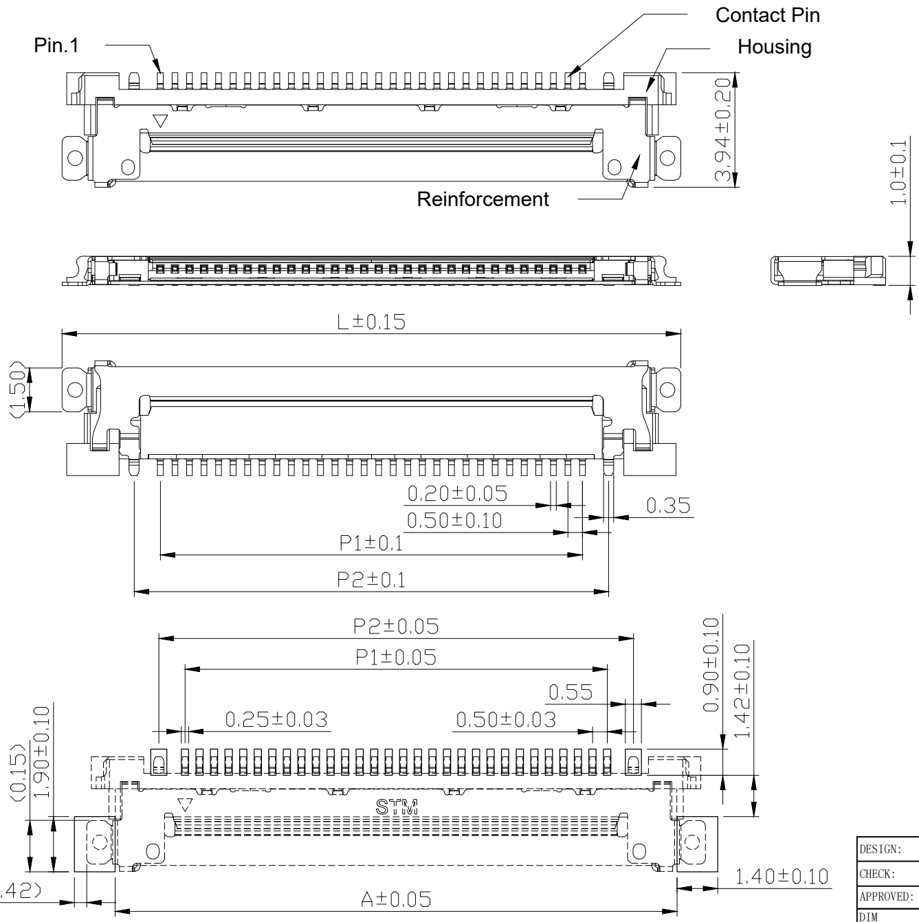
P.C.B LAYOUT
